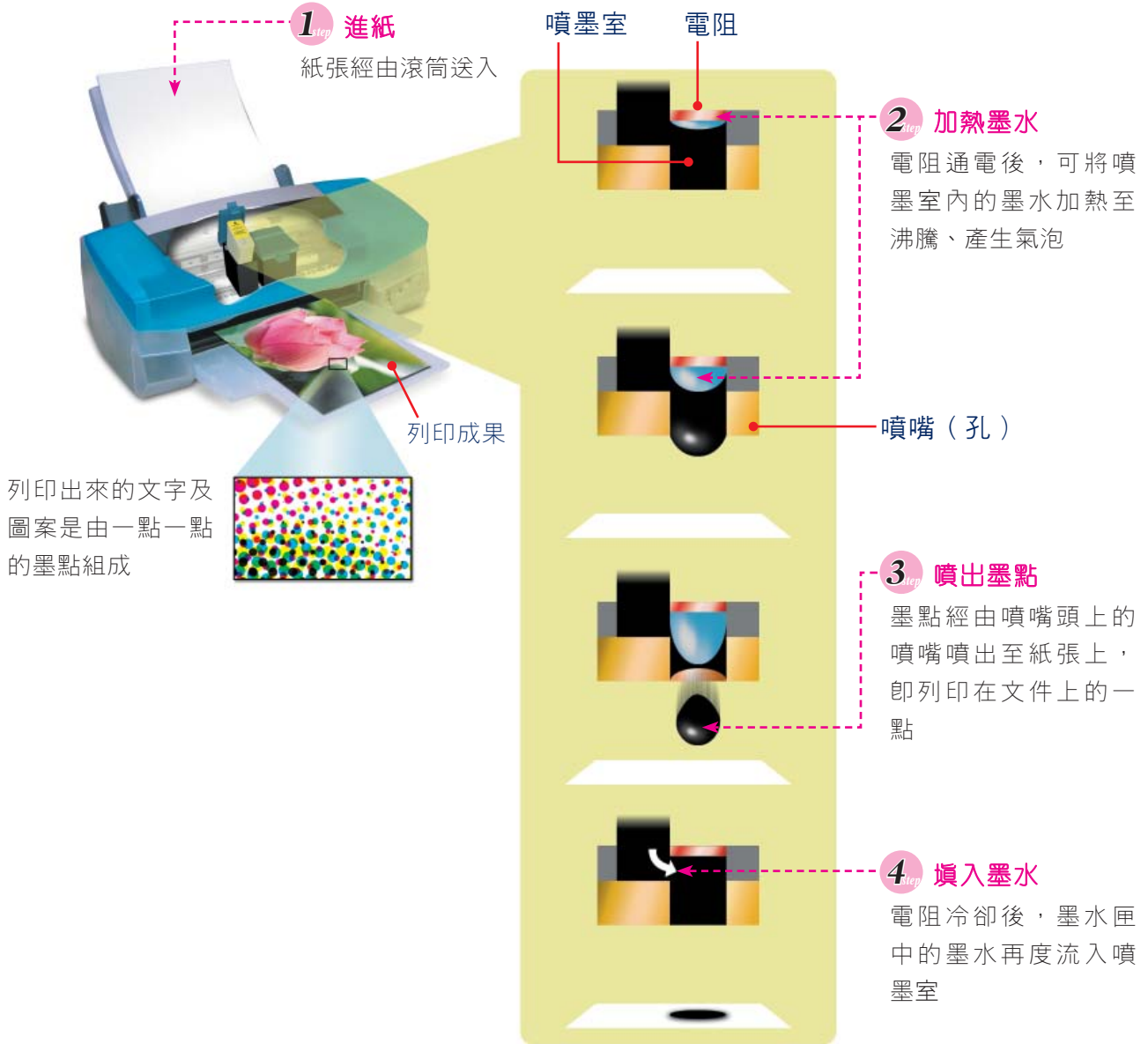
圖5-33 噴墨印表機的工作原理
