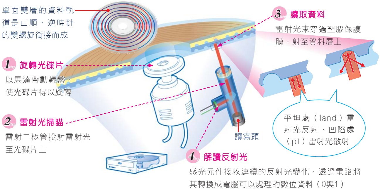
圖5-11 DVD光碟機的工作原理
