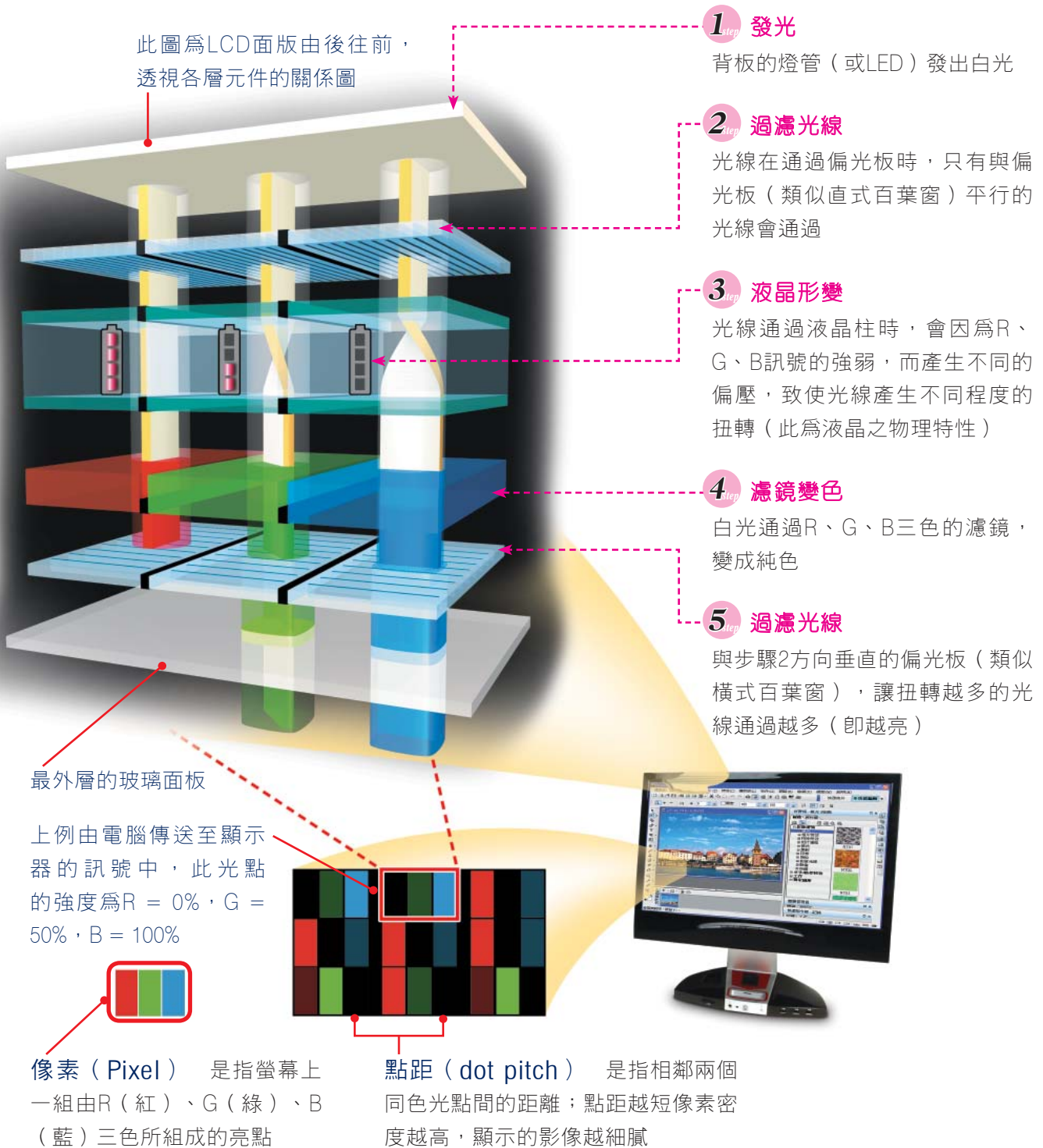
圖5-26 LCD呈像原理
