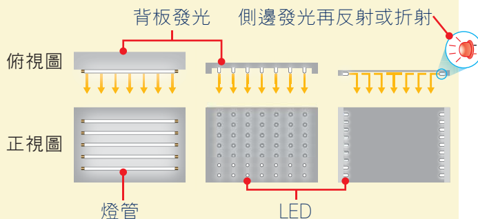
圖5-25 燈管 vs. LED背光源
