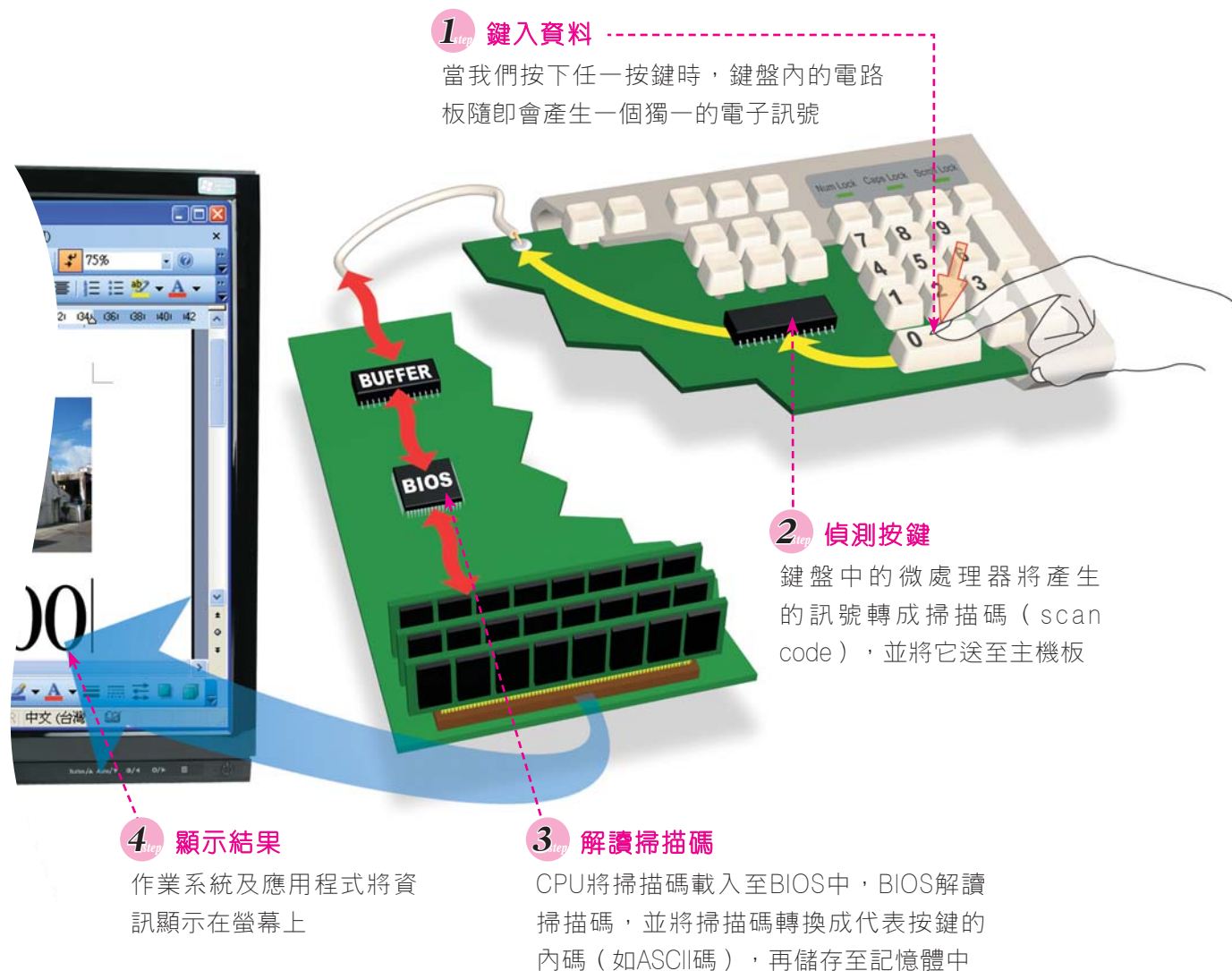
圖5-14 鍵盤的工作原理
