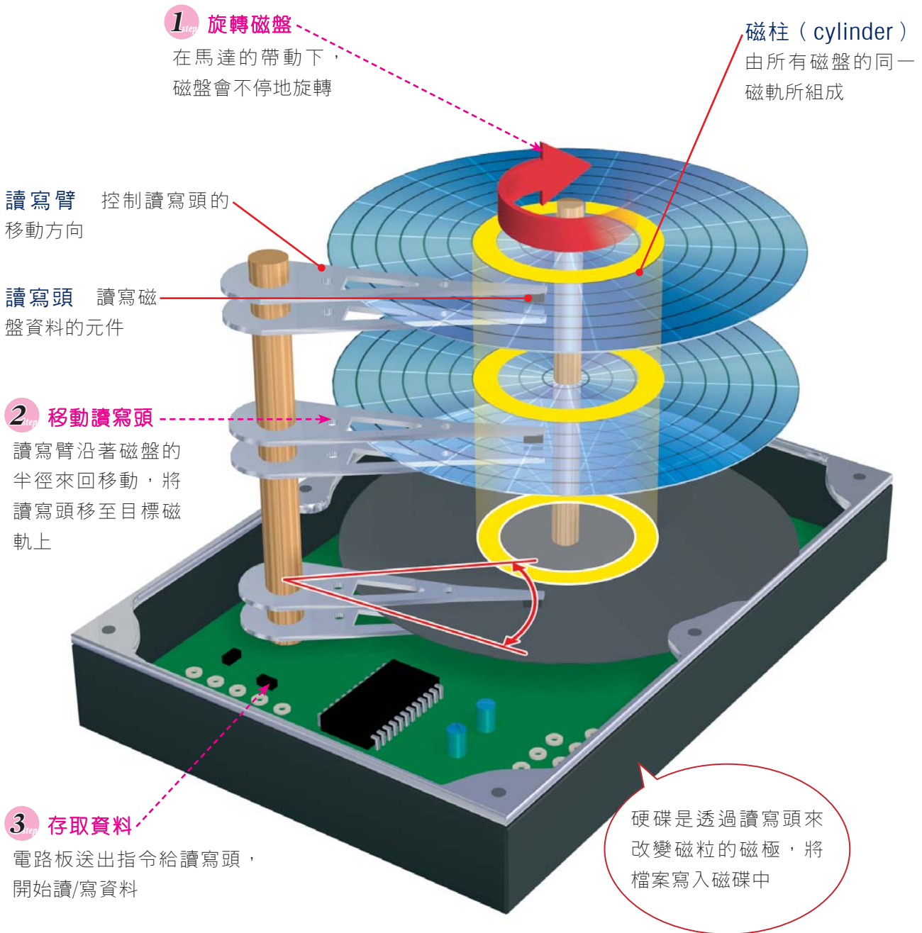
圖5-7 硬碟的內部結構與讀寫原理
