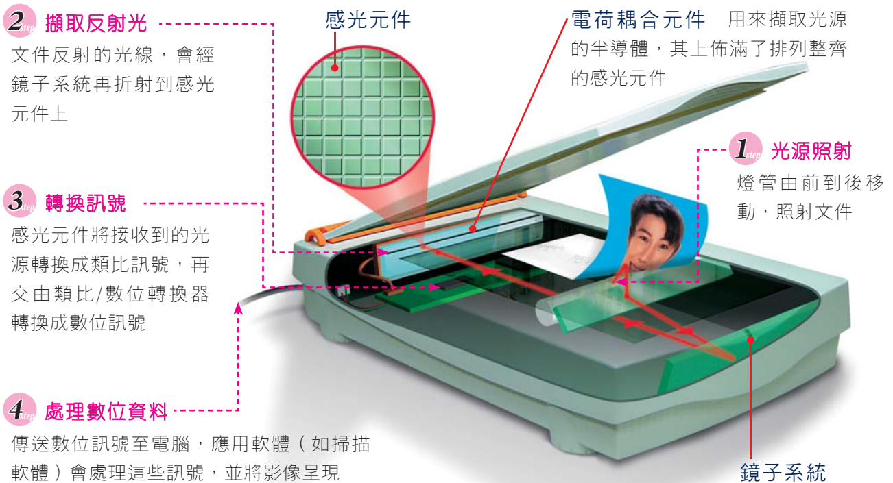
圖5-19 平台式掃描器的工作原理
